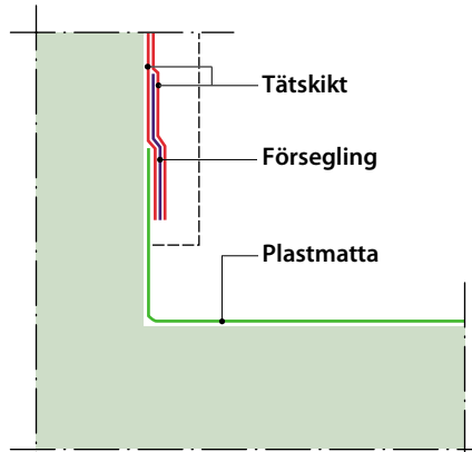
FIGUR 11. Anslutning mot plastmatta, golv.
