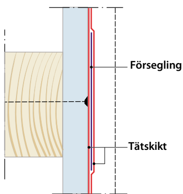
FIGUR 9. Skruvrad i skivvägg.
